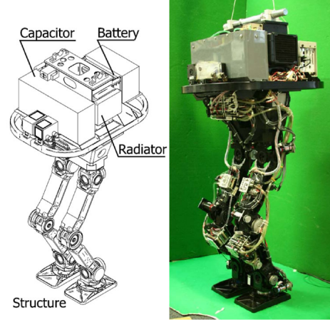
d) U. Tokyo HRP3La-JSK motor
