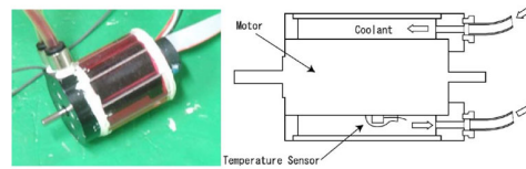
d) U. Tokyo HRP3La-JSK motor
