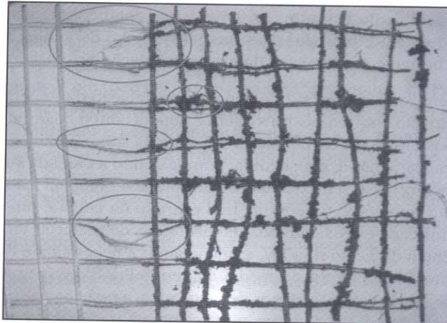
Fig. 8 – Geogrelha de fibra de vidro com ruptura em vários pontos após ensaio de arrancamento com solo argiloso (subleito) na camada inferior e pedregulho areno-siltoso (base) na camada superior, sobrecarga de 21 kPa.
