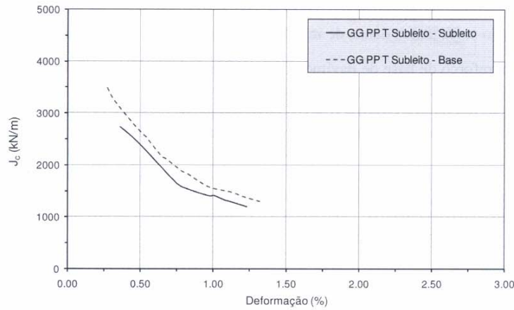
Fig. 10 – Curvas Rigidez x Deformação dos Ensaio 2 e 4 (sobrecarga 21 kPa). Nota: GG – Geogrelha; PP – Polipropileno; T – Transversal (sentido de fabricação).
