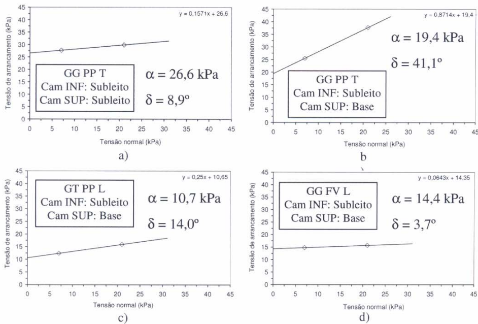
Fig. 11 – Envolvórias dos ensaios de arrancamento. a) Ensaio 1 e 2. b) Ensaio 3 e 4. c) Ensaio 5 e 6. d) Ensaio 7 e 8.
