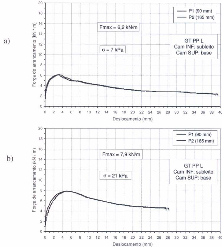
Fig. 6 – Curvas Força x Deslocamento. a) Ensaio 5. b) Ensaio 6. Nota: F_{max} – Força de Arrancamento Máxima; s - Sobrecarga; Cam – Camada; INF – Inferior; SUP – Superior; GT – Geotêxtil; PP – Polipropileno; L – Longitudinal (sentido de fabricação); Números entre parêntesis - distância do ponto em relação à parede frontal da caixa de arrancamento.
