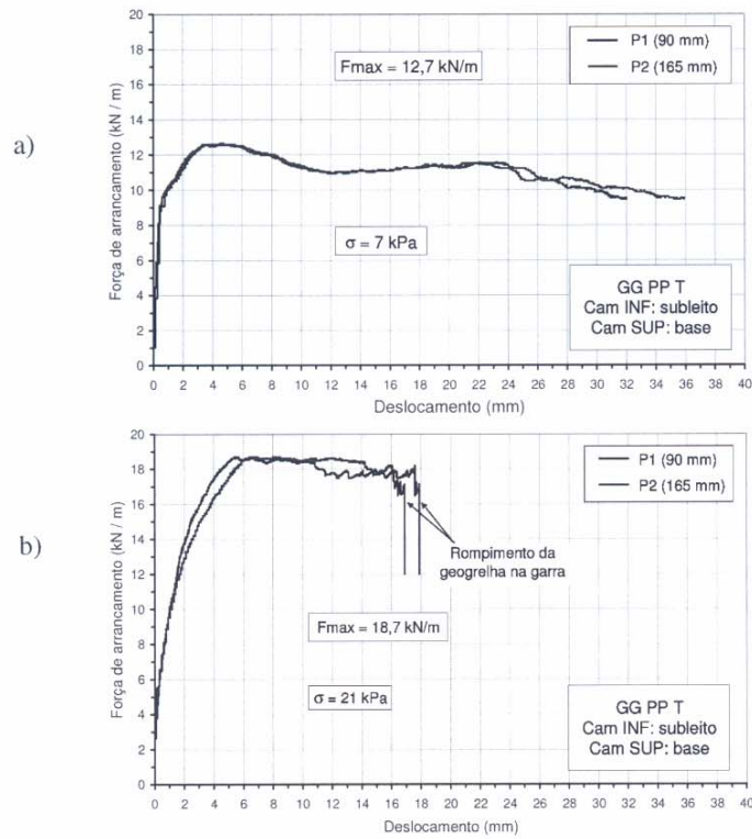
Fig. 5 – Curvas Força x Deslocamento. a) Ensaio 3. b) Ensaio 4. Nota: F_{\max} – Força de Arrancamento Máxima; s - Sobrecarga; Cam – Camada; INF – Inferior; SUP – Superior; GG – Geogrelha; PP – Polipropileno; T – Transversal (sentido de fabricação); Números entre parêntesis - distância do ponto em relação à parede frontal da caixa de arrancamento.
