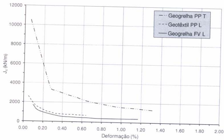
Fig. 9 – Curvas Rigidez Confinada ( J_c ) x Deformação dos Ensaios 4, 6 e 8 (sobrecarga 21 kPa). Nota: T – Transversal (sentido de fabricação); L – Longitudinal (sentido de fabricação); PP – Polipropileno; FV – Fibra de vidro.
