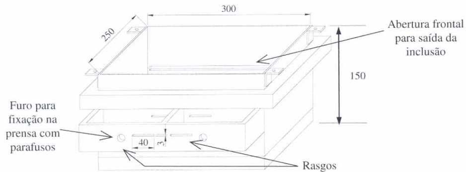
Fig. 1 – Perspectiva da caixa de pequenas dimensões para ensaios de arrancamento. Dimensões em mm.
