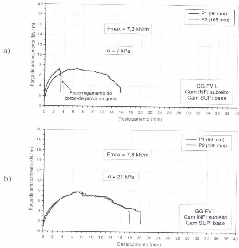
Fig. 7 – Curvas Força x Deslocamento. a) Ensaio 7. b) Ensaio 8. Nota: F_{max} – Força de Arrancamento Máxima; s - Sobrecarga; Cam – Camada; INF – Inferior; SUP – Superior; GG – Geogrelha; FV – Fibra de Vidro; L – Longitudinal (sentido de fabricação); Números entre parêntesis - distância do ponto em relação à parede frontal da caixa de arrancamento.
