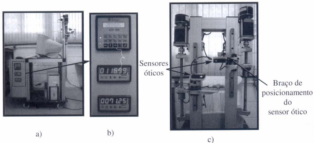
Fig. 2 – Medidor de deslocamentos a laser e seus componentes. a) Vista geral do equipamento. b) Controlador Lógico Programável (CLP) e contadores. c) Sensores óticos e braços de posicionamento dos sensores óticos.
